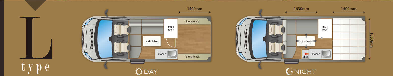
ダブルベッドタイプ 乗車定員：5名 就寝定員：2名＋子供1名
