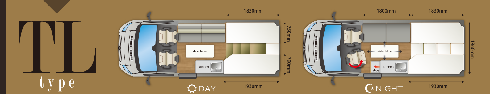
乗車定員：6名 就寝定員：2名 中央マット使用時／4名
