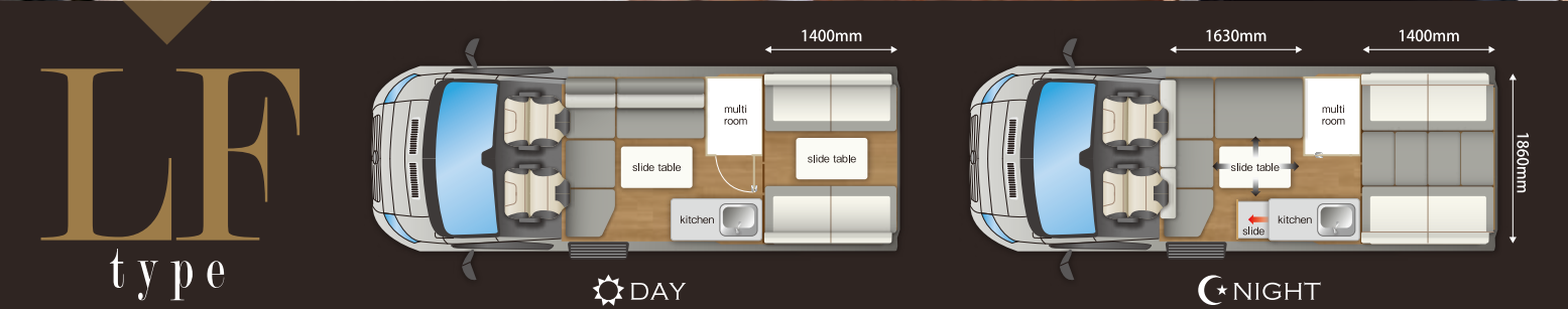
フルダウンベッドタイプ 乗車定員：7名 就寝定員：4名＋子供1名
